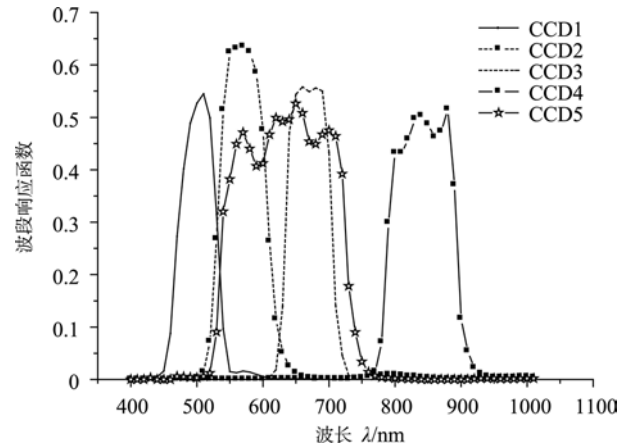
图 1 CBERS02B 星 CCD 传感器的波段响应函数
