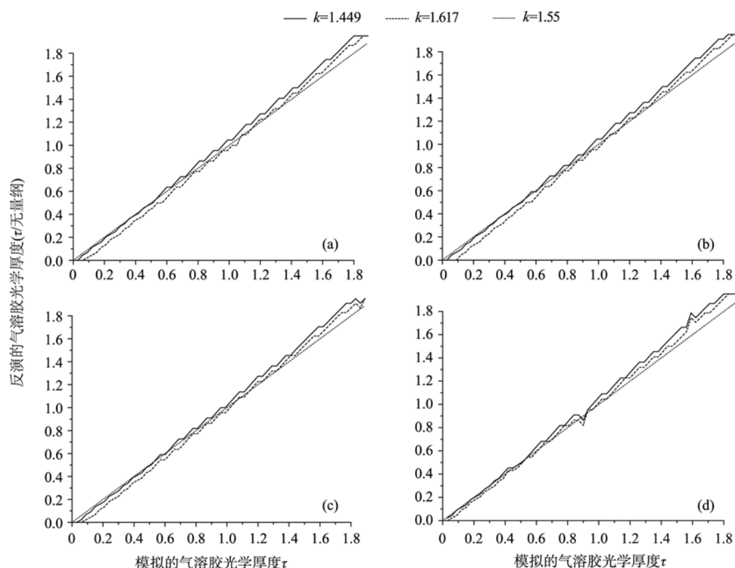
图5 红蓝波段地表反射率比率误差对气溶胶反演的影响
